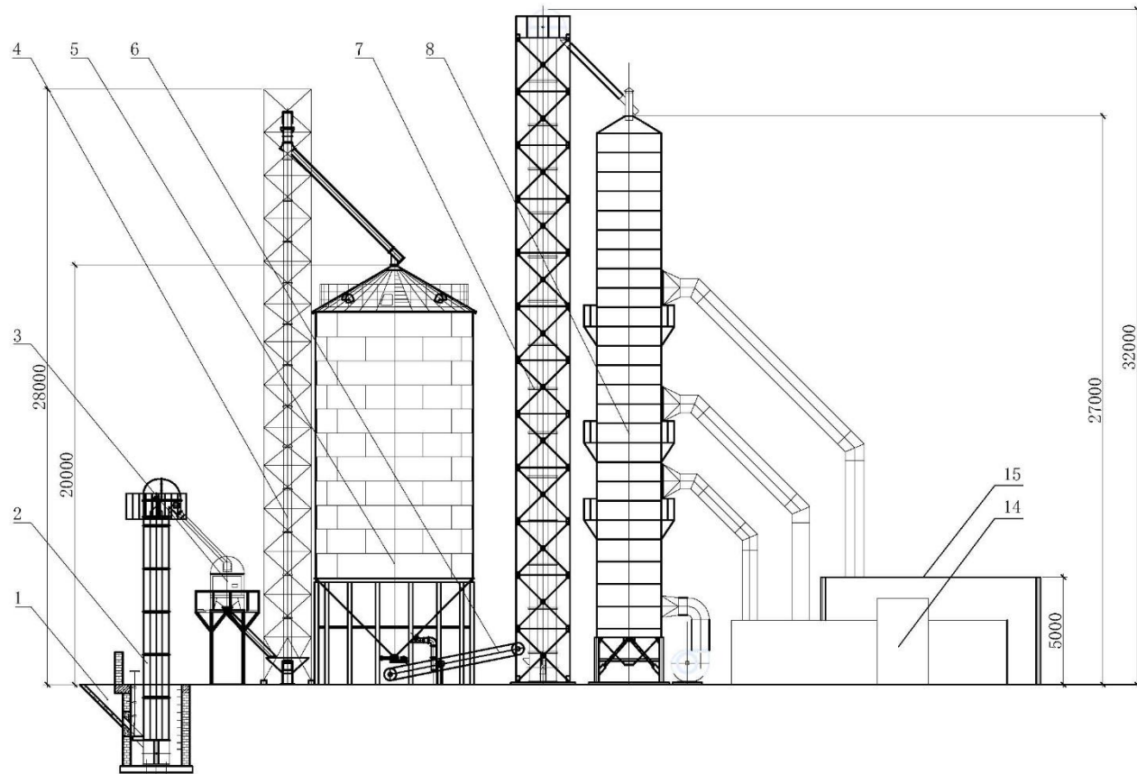
1.卸粮斗 2.1#提升机 3.初清筛 4.2#提升机 5.烘前仓 6.1#皮带输送机 7.3#提升机 8.连续式干燥机 14.燃气换热器 15.热风炉间
